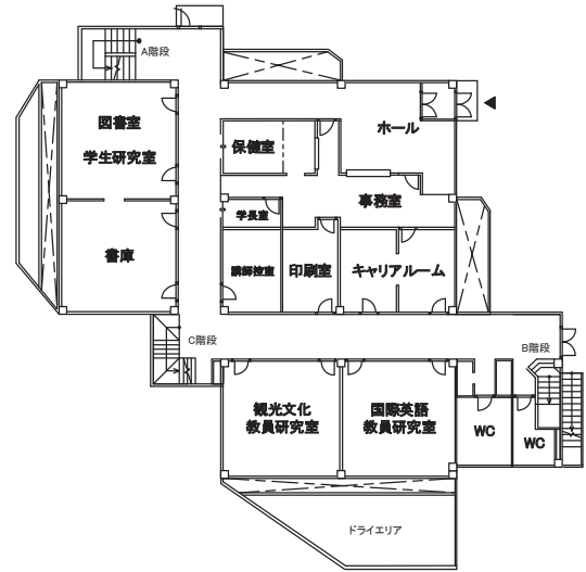
3階
