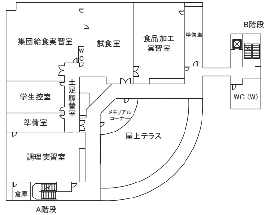
4階
